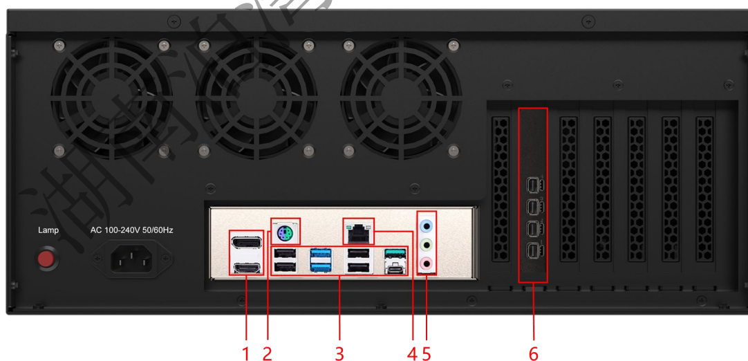
设备背面图
