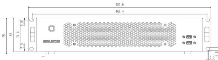
正视图
