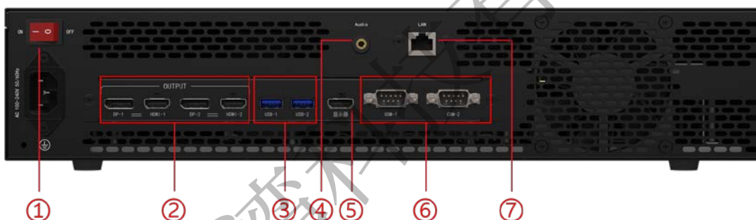
设备背面图
